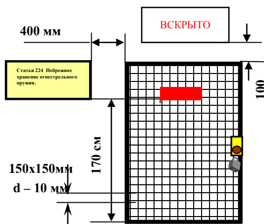
Рис. 3 Оборудование входной двери в КХО
